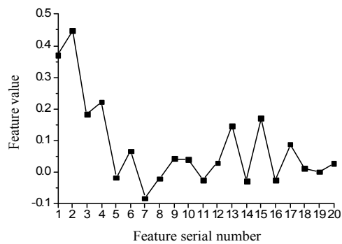
(d) Feature values (no rubbing)
